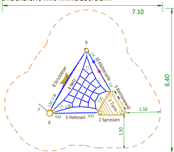
Draufsicht mit Mindestraum
