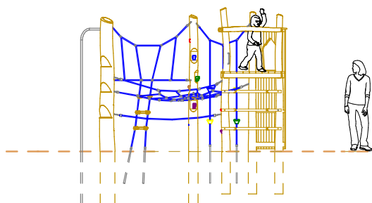
Ansicht
